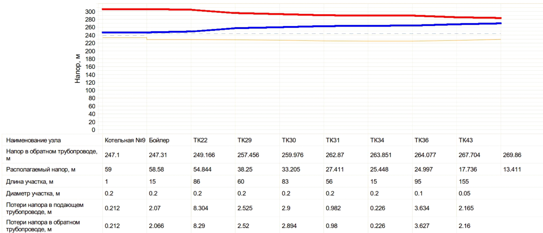
Рисунок 7 - Пьезометрический график тепловой сети от Котельной №9 до определяющего потребителя – административное здание (ул. Пионерская, 19)
