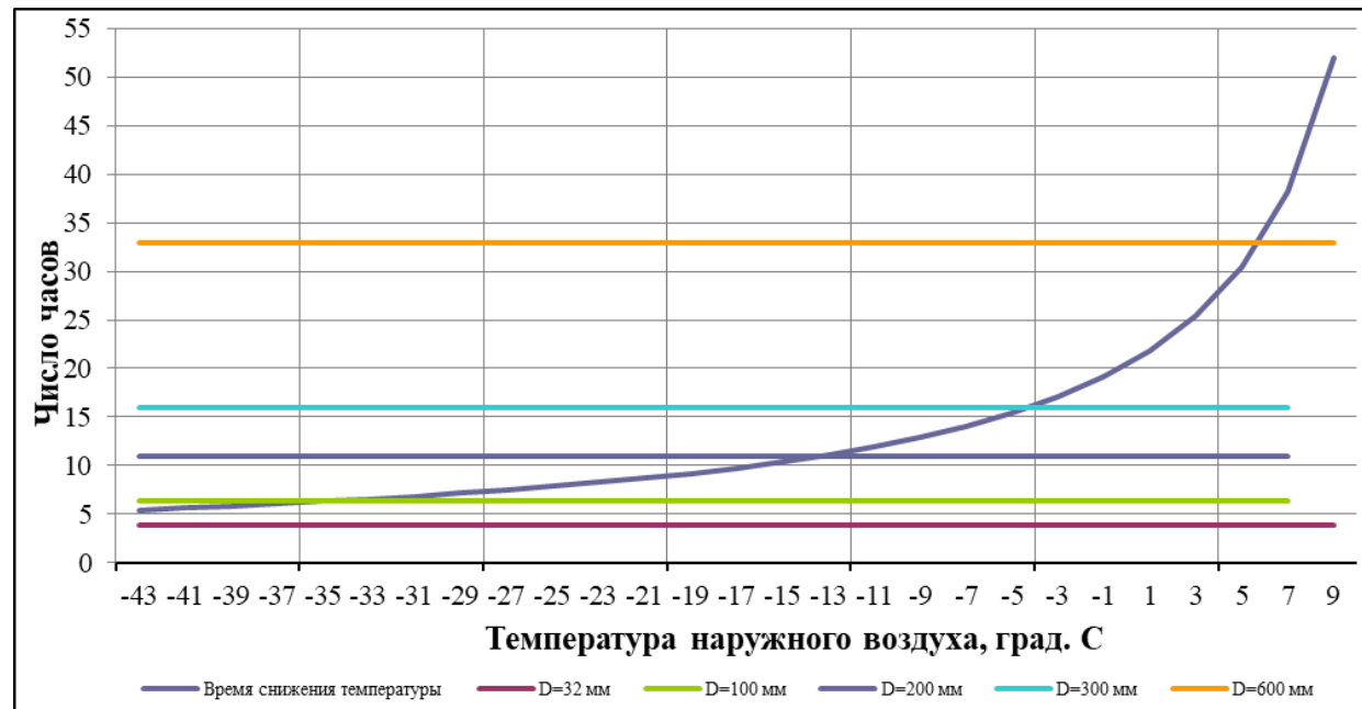
Рисунок 16 - Графическое сравнение периода времени снижения температуры внутреннего воздуха до критического значения и периода времени, необходимого для восстановления участка тепловой сети
