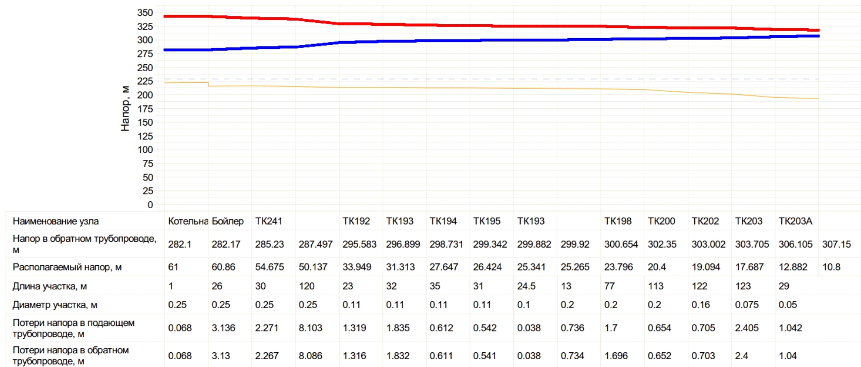
Рисунок 12 - Пьезометрический график тепловой сети от Котельной №27 до определяющего потребителя – жилой дом (ул. С.Сайдашева, 32)
