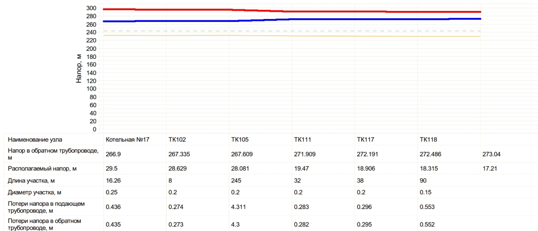
Рисунок 10 - Пьезометрический график тепловой сети от Котельной №17 до определяющего потребителя – административное здание (ул. Пионерская, 9)
