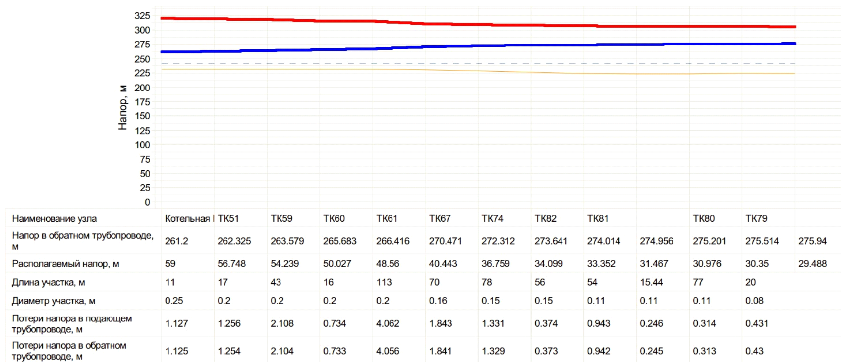
Рисунок 8 - Пьезометрический график тепловой сети от Котельной №10 до определяющего потребителя – жилой дом (ул. Пушкина, 31)
