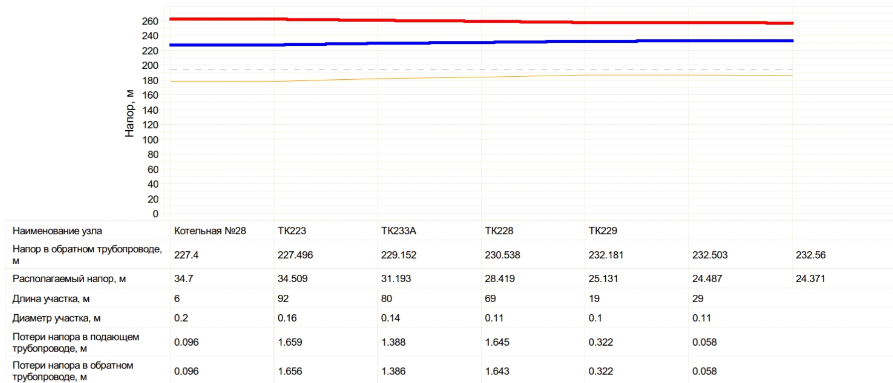
Рисунок 13 - Пьезометрический график тепловой сети от Котельной №28 до определяющего потребителя – Жилой дом (ул. Калинина, 46)
