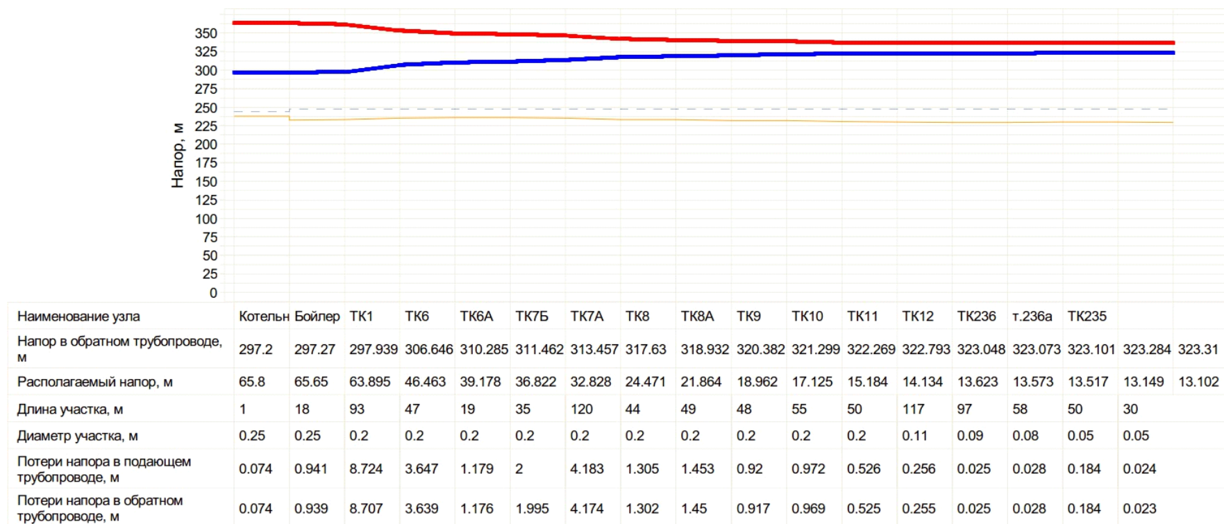
Рисунок 9 - Пьезометрический график тепловой сети от Котельной №15 до определяющего потребителя – нежилое здание (ул. С.Сайдашева д. б/н)
