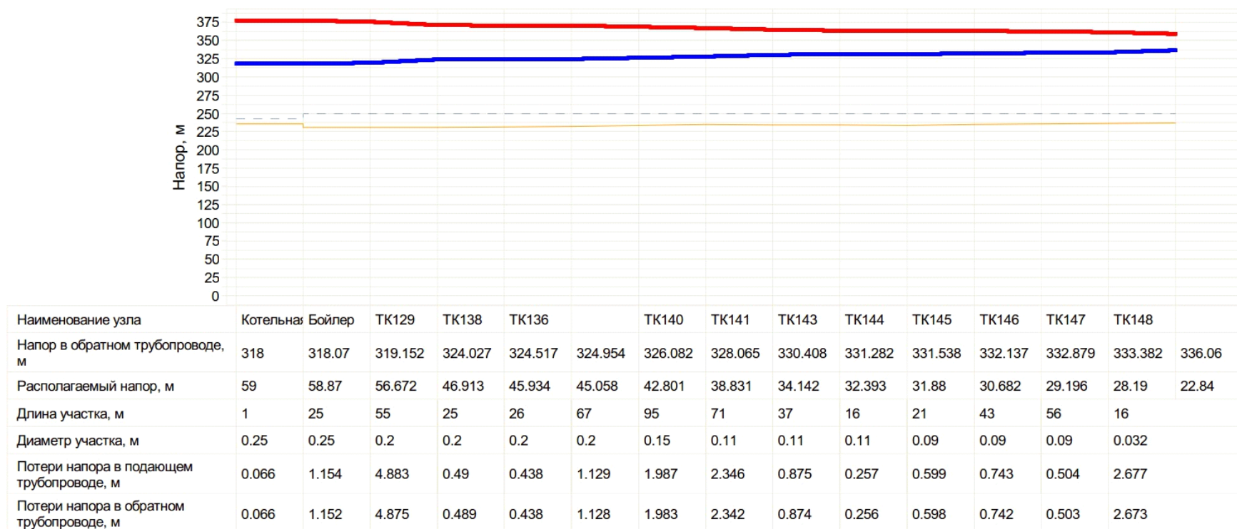
Рисунок 11 - Пьезометрический график тепловой сети от Котельной №23 до определяющего потребителя – административное здание (ул. Пионерская, 9)
