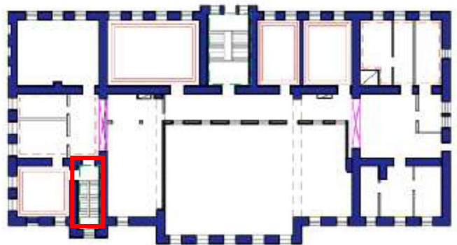
38 нче рәсем. Кара (икенче дәрәжә) баскычның урнашу урынын күрсәтеп, ике катлы күләмнең беренче каты схемасы (Литер А)
