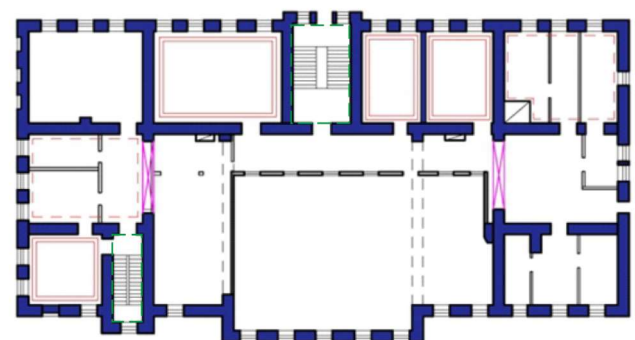
5 нче рәсем. Подвалның чын элементлары схемасы (ике катлы күләм, литер А)
