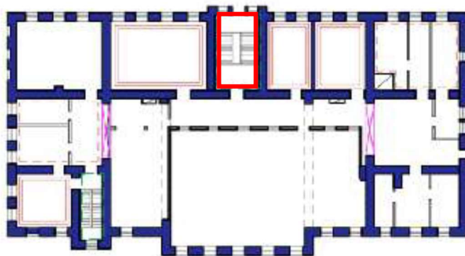
34 нче рәсем. Парад баскычының урынын күрсәтеп, ике катлы күләмле беренче кат схемасы (Литер А)
