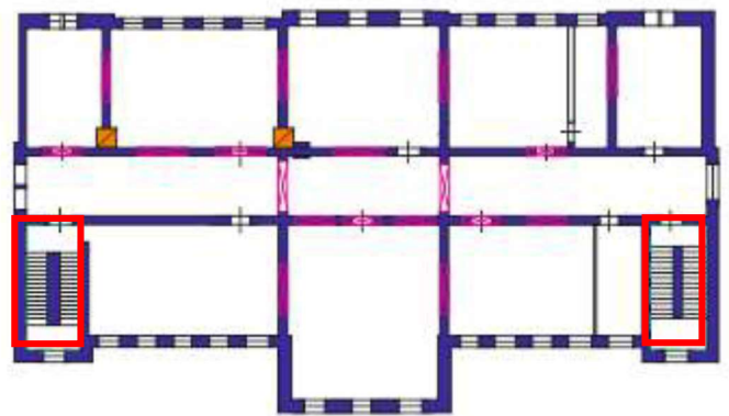
41 нче рәсем. Баскычларның урнашу урынын күрсәтеп, өч катлы күләмнең беренче каты схемасы (Литер А1)
