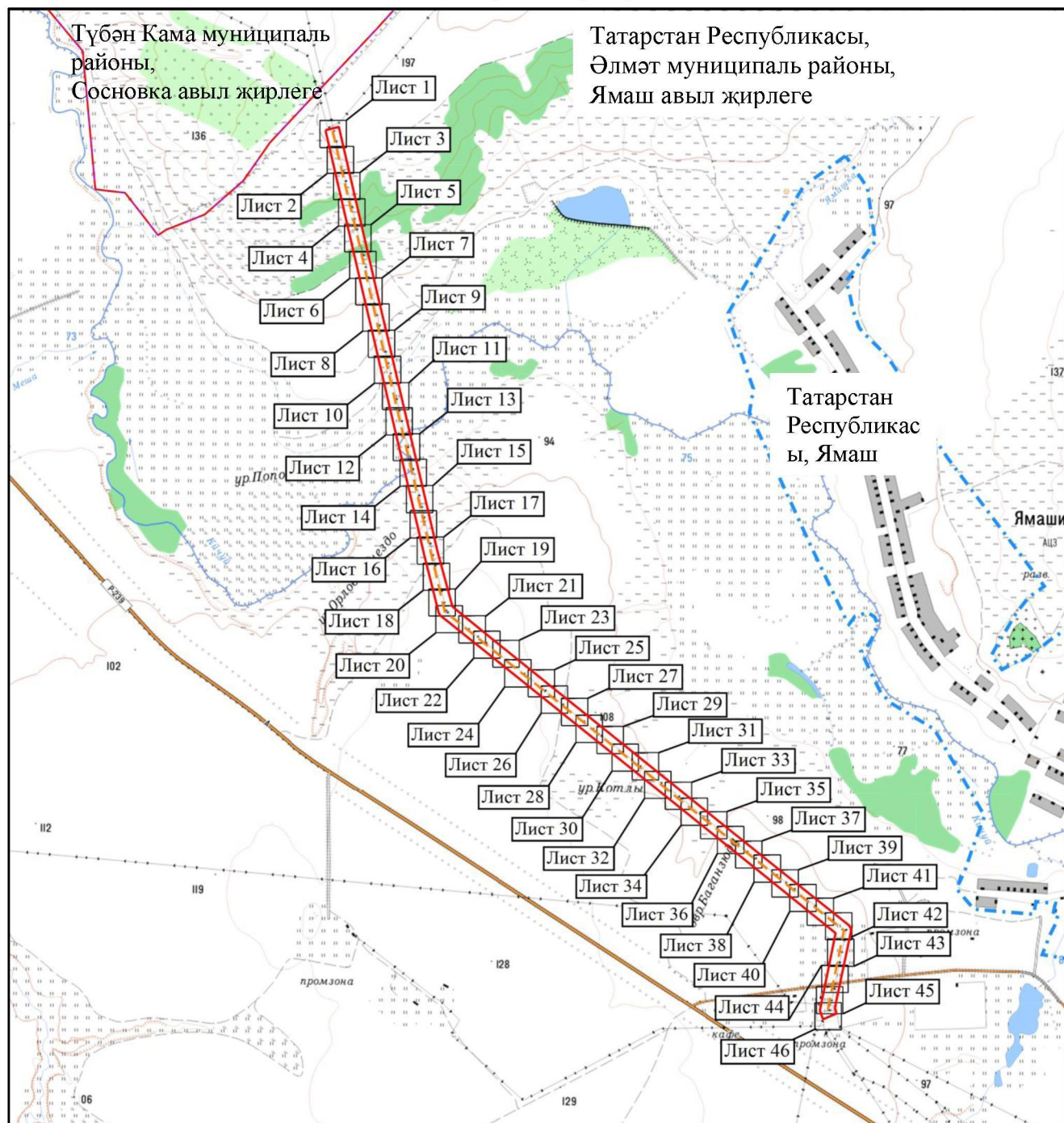
Объект чикләренә күзәтү схемасы
