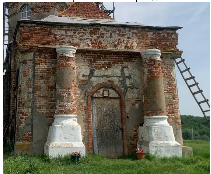
4 нче рәсем. Манараның көнбатыш фасады
