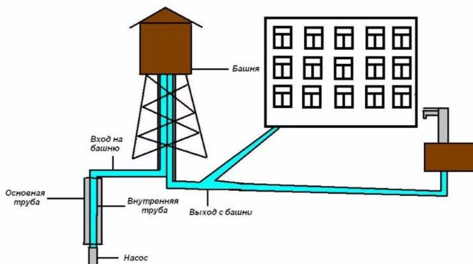
Рәсем 2 – Принципиаль схемасы су башка су башнясы (1 – чыганагы, су белән тээмин итү, скважина; 2 – кулланучылар)
