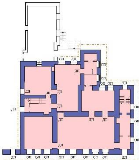
17 нче рәсем. Беренче кат планы
