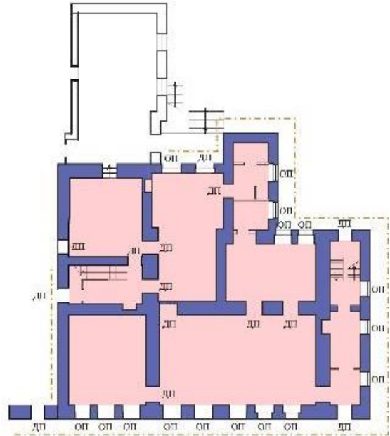
4 нче рәсем. Беренче кат планы
