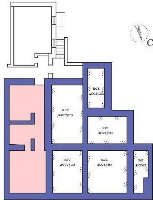
20 нче рәсем. Подвал катының планы
