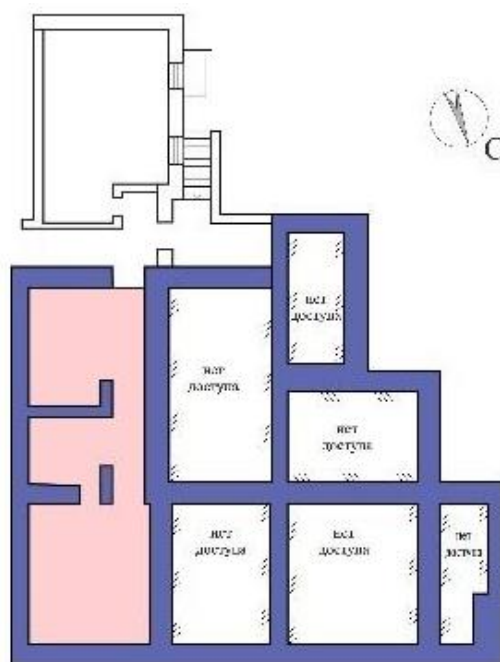
30 нчы рәсем. Подвал катының планы
