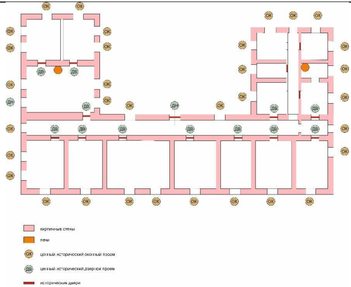
5 нче рәсем. Конструктив схема
