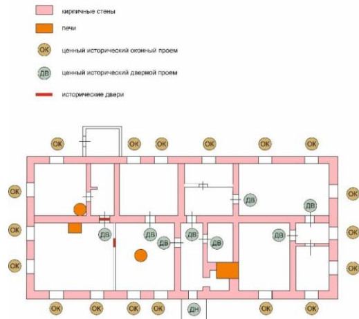
4 нче рәсем. Конструктив схема
