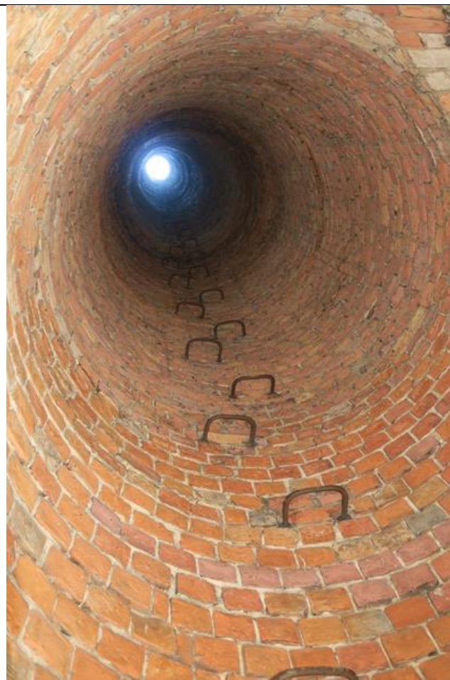
17 нче рәсем. Кладкадагы тимер кыстыргычлар
