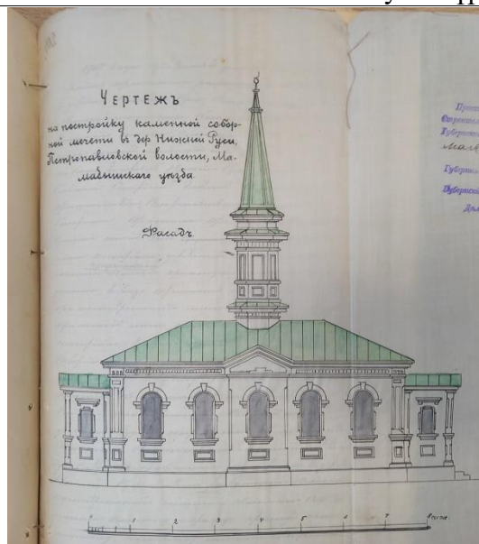
Рәсем. 4. Түбән Үрәс авылында мәчет төзү өчен архив проекты, 1907 ел
