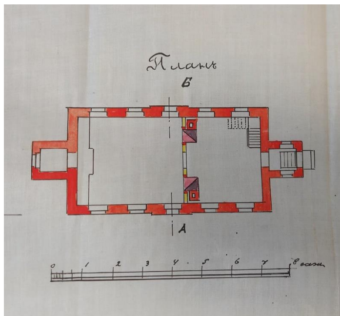
Рәсем. 5. Түбән Үрәс авылында мәчет төзү өчен архив проекты, 1907 ел
