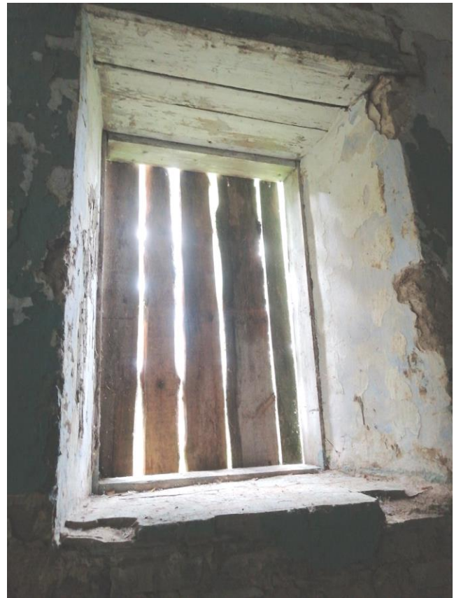
Рәсем. 29. Тәрзә уемнарының аркылы агач такталары
