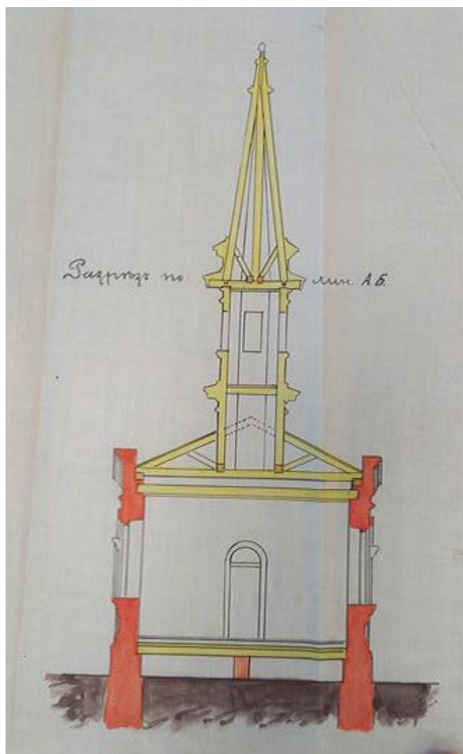
Рәсем. 18. Чатыр төсле тәмамланган күпкырлы манараның урнашу урыны, габаритлары, конфигурациясе
