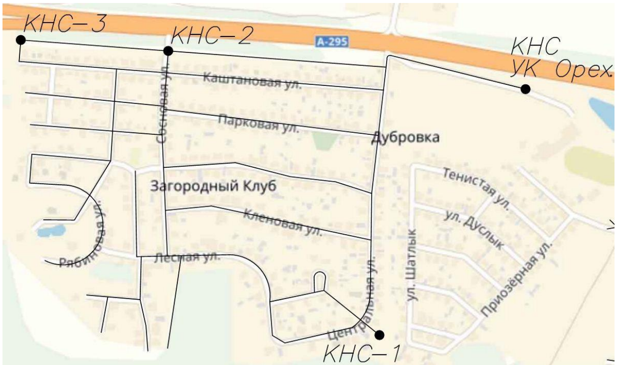
Дөге.2 Үзәк Ореховка һәм коттедж бистэләренең ташландык суларны агызу схемасы Көнбатыш Ореховка
