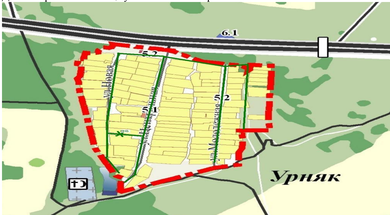
Дөге.7. Үрнәк авылының су белән тәмин итү схемасы
