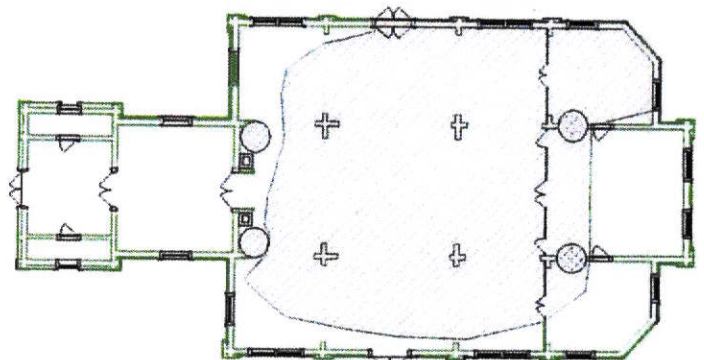
Рис. 12. Схема перекрытий
