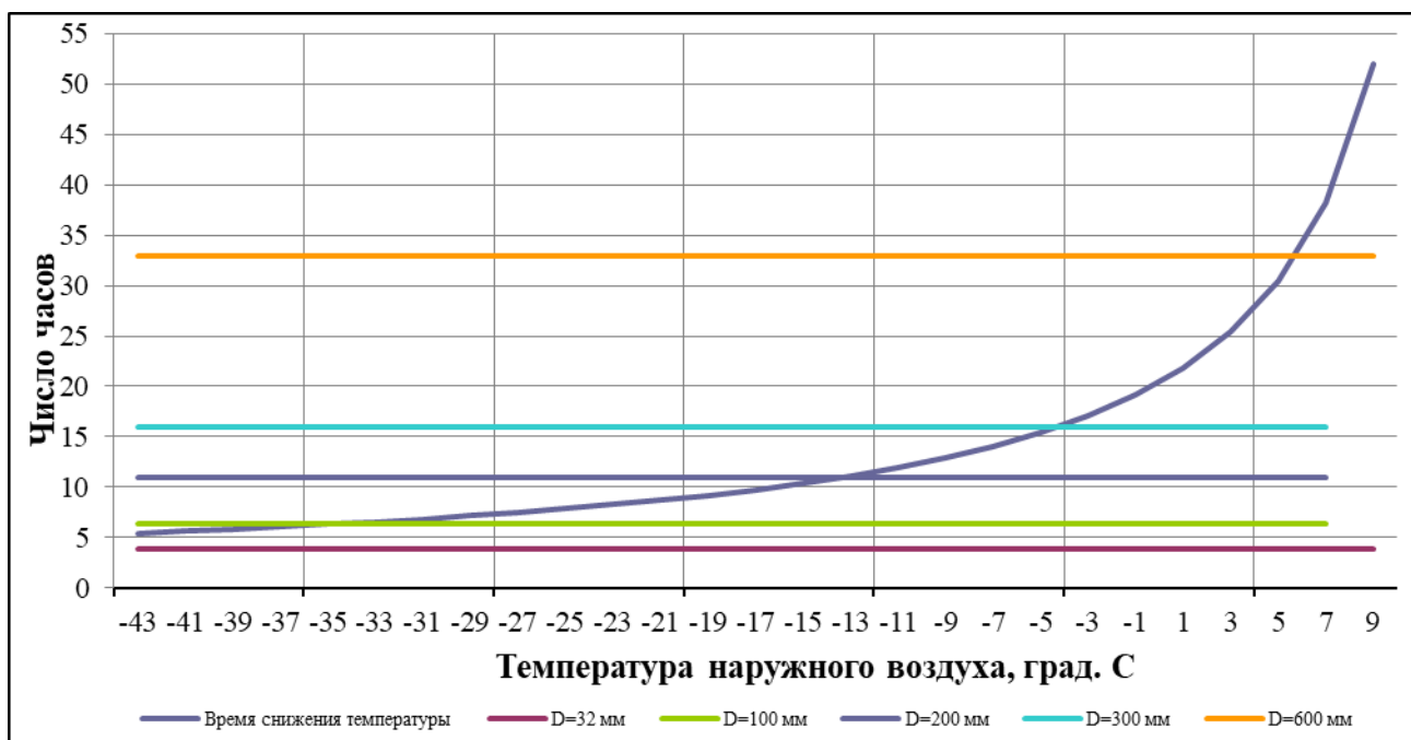
Рисунок 8 - Графическое сравнение периода времени снижения температуры внутреннего воздуха до критического значения и периода времени, необходимого для восстановления участка тепловой сети.
