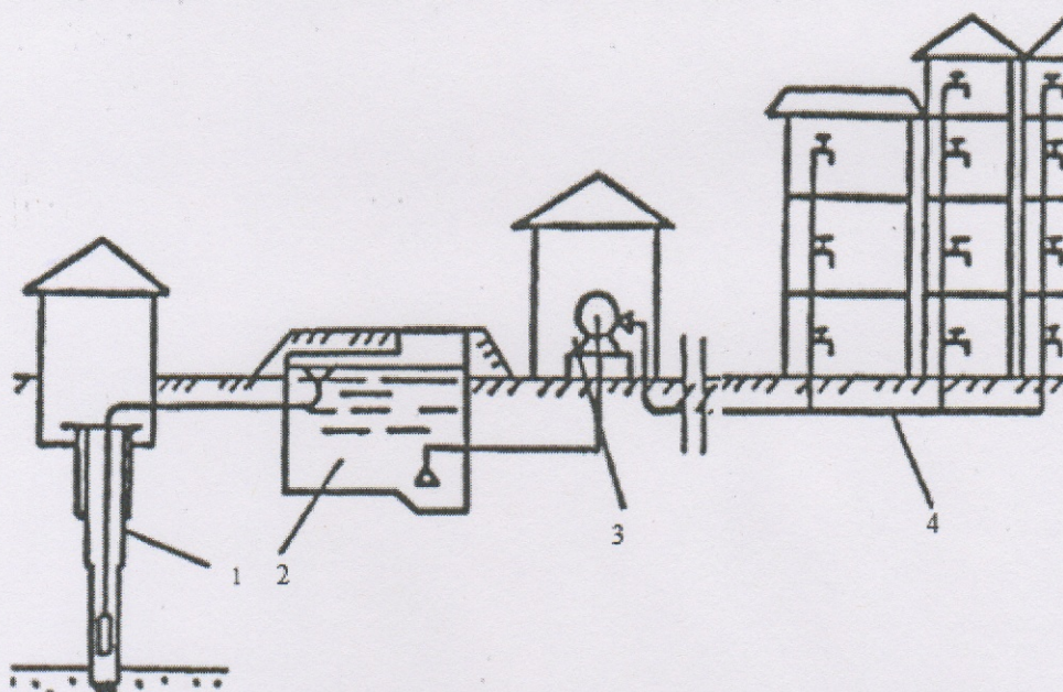
Рисунок 1 – Принципиальная схема водоснабжения (1 – источник водоснабжения; 2 – резервуар чистой воды; 3 – насосная станция; 6 – потребители)
