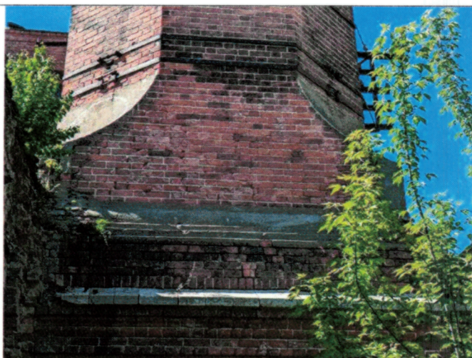
Рис. 12. Вставки белого камня у основания трубы
