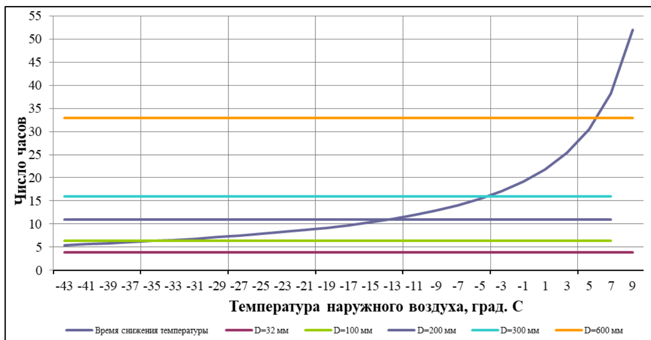
Рисунок 11.2 - Графическое сравнение периода времени снижения температуры внутреннего воздуха до критического значения и периода времени, необходимого для восстановления участка тепловой сети
