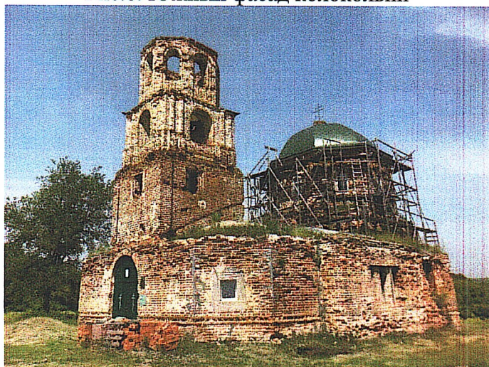
Рис.7. Восточный фасад
