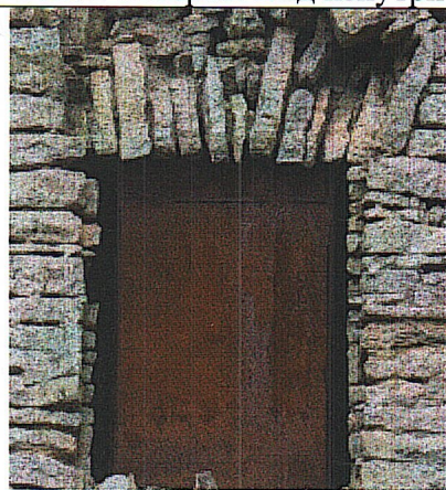
Рис.5. Лучковые перемычки оконных проемов
