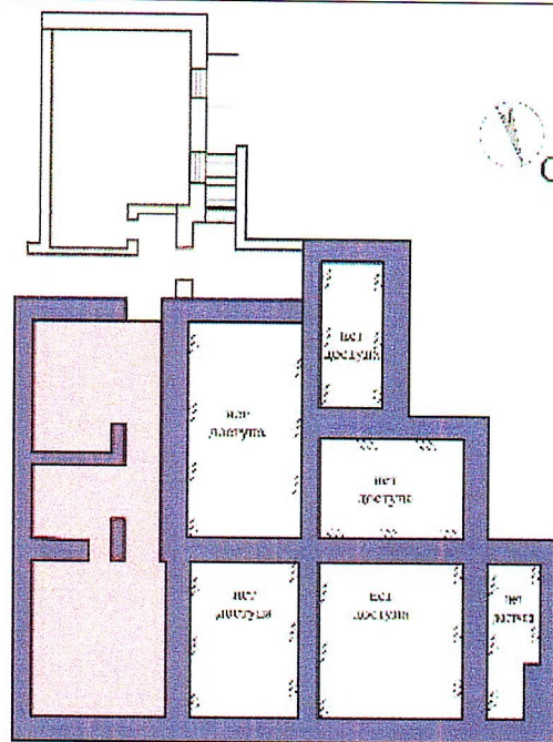
Рис. 20. План подвального этажа
