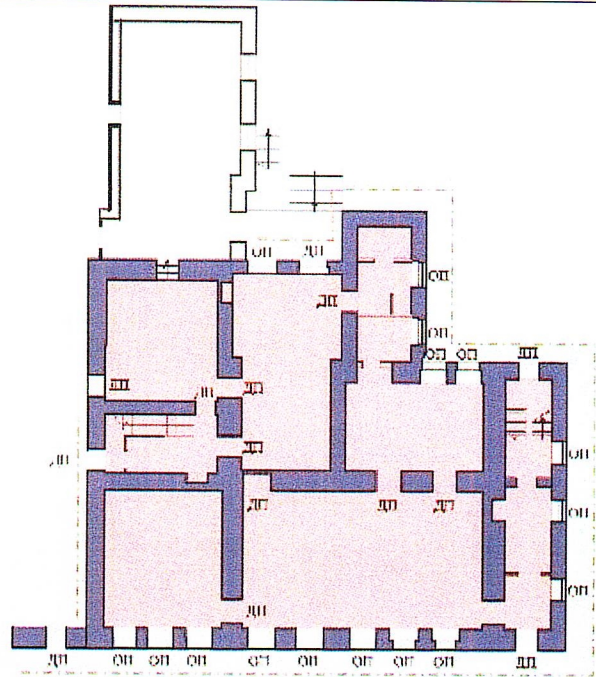
Рис.17. План первого этажа
