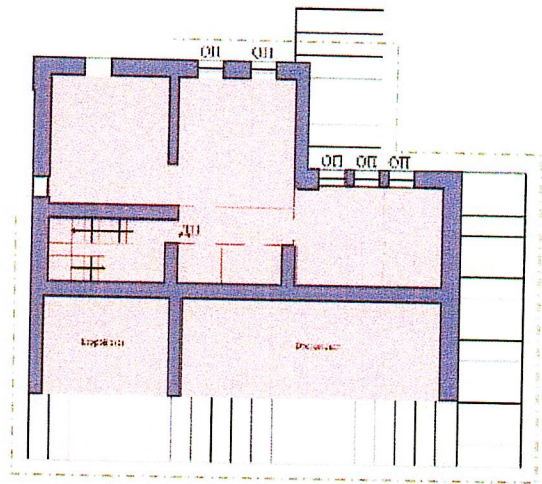
Рис.29. План антресольного этажа
