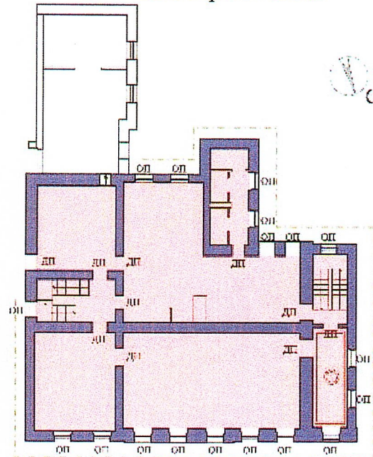
Рис.5. План второго этажа
