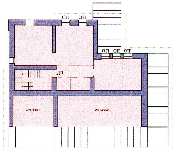
Рис.19. План антресольного этажа
