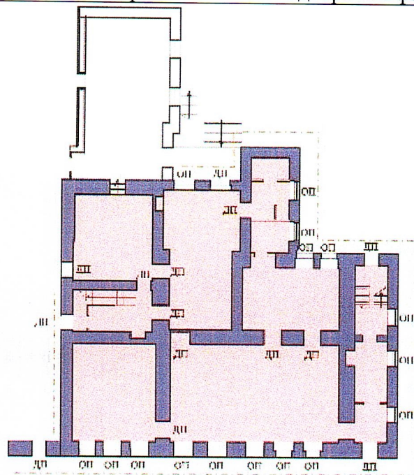
Рис.27. План первого этажа
