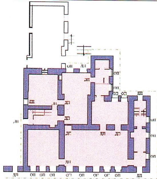
Рис.4. План первого этажа
