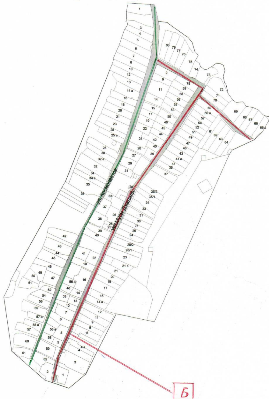
СХЕМА водоснабжения деревни Сарайлы
