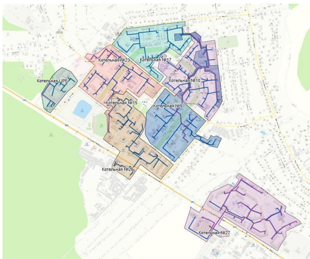
Рисунок 5 – Зоны теплоснабжения Котельной №9, Котельной №10, Котельной №15, Котельной №17, Котельной №23, Котельной №26, Котельной №27, Котельной ЦРБ
